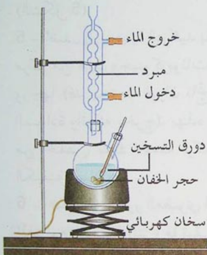
التركيب التجريبي
