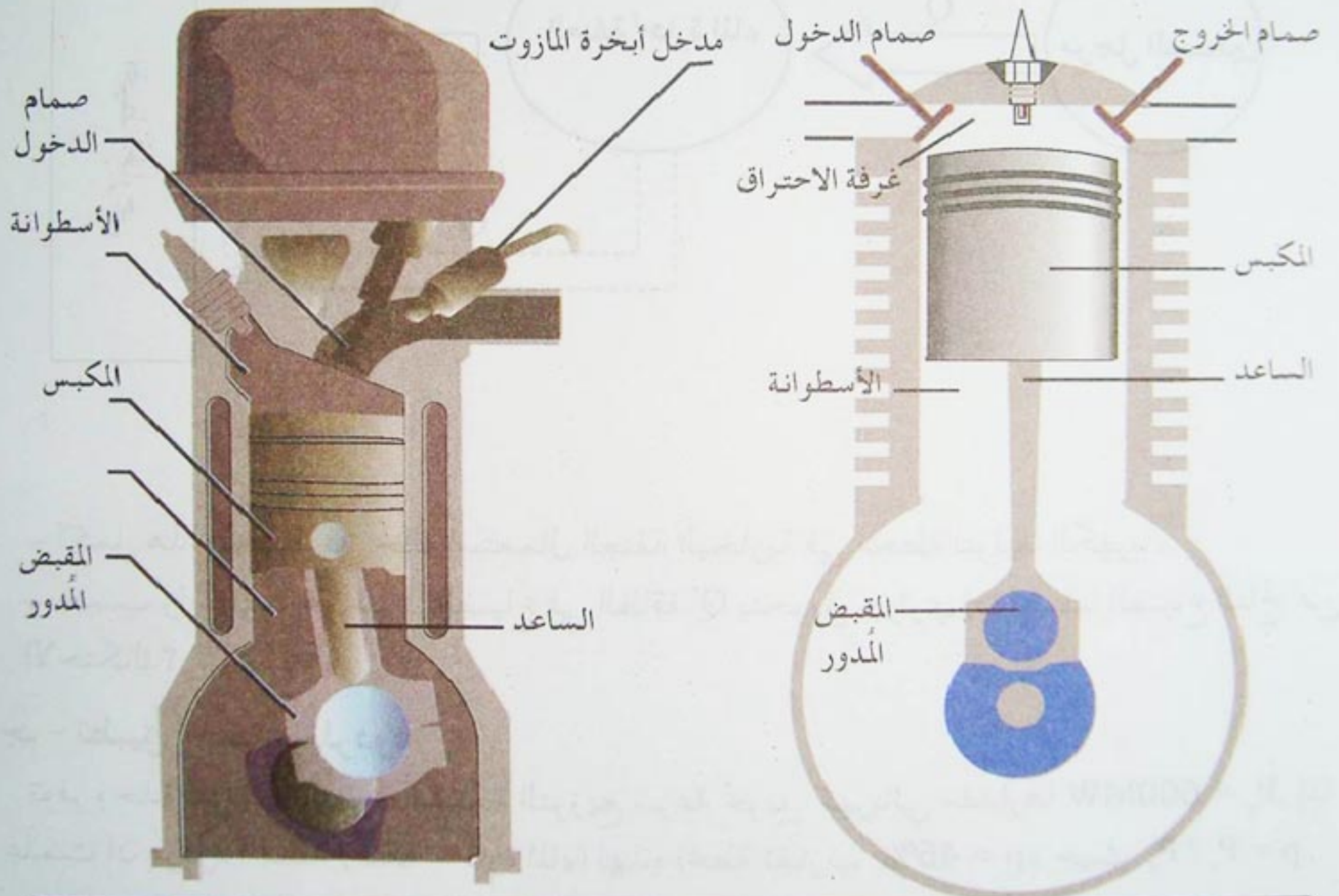
(الشكل 2): مخطط غرفة الاحتراق لمحرك ديازل
