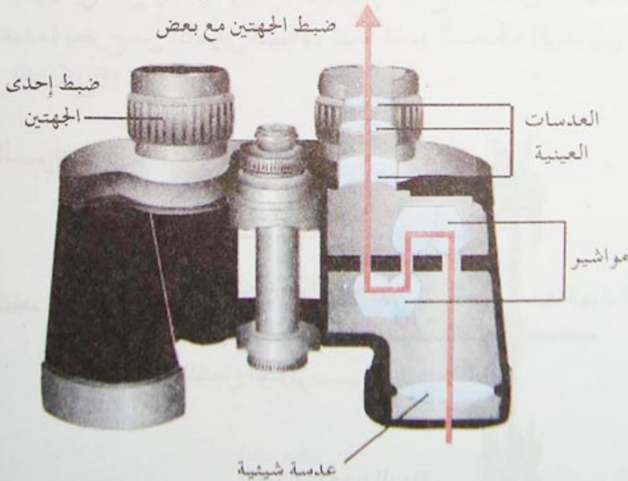
(الشكل 4) : مسار شعاع ضوئي داخل المنظار الموشوري
