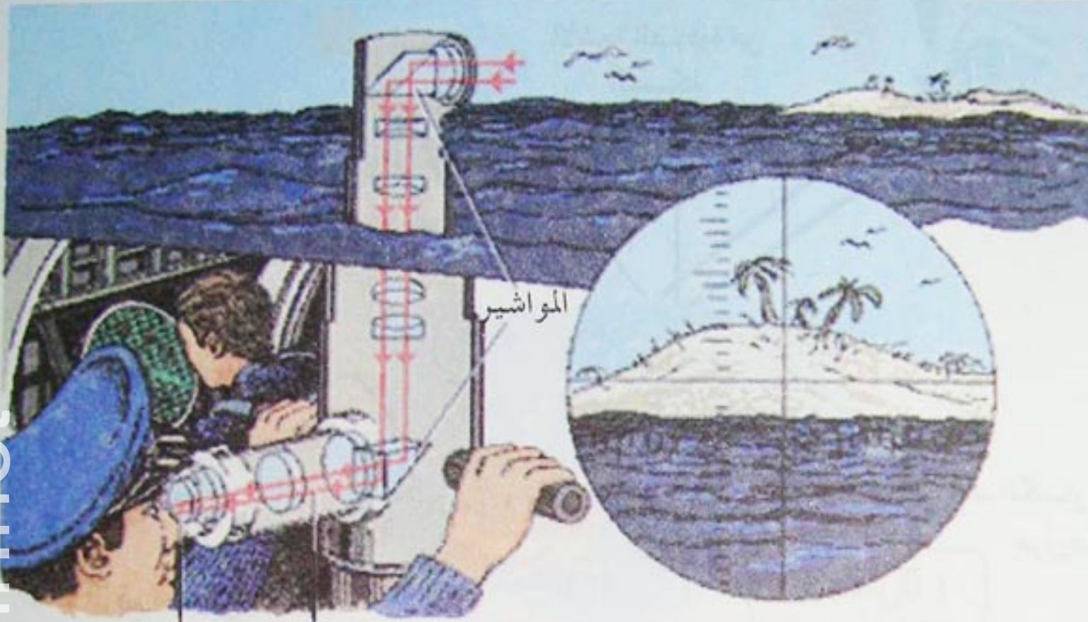
(الشكل 3) : منظار الأفق الموشوري
