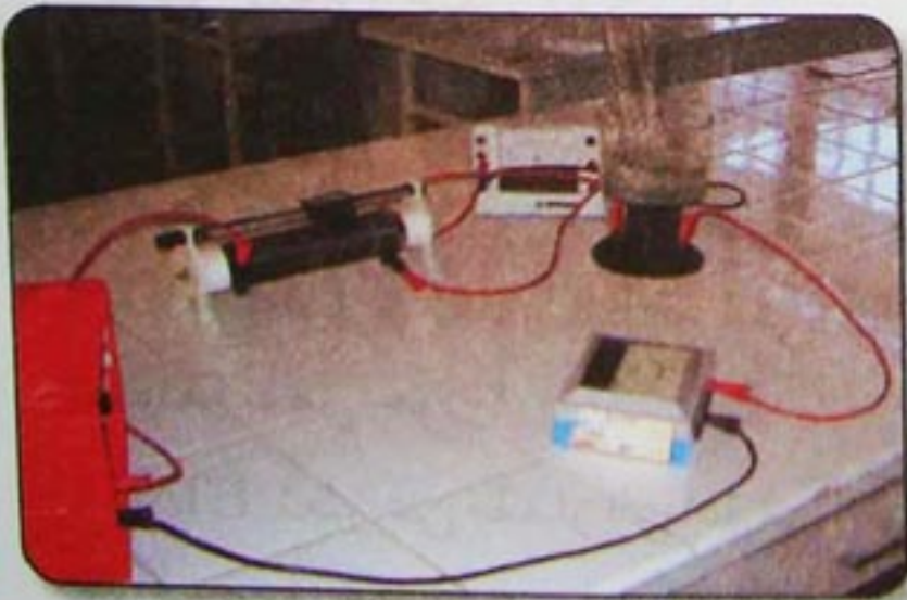
التركيب التجريبي
